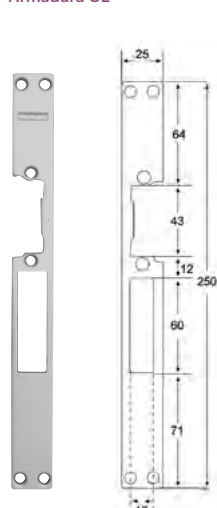
Armadura GE
