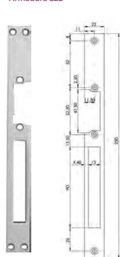
Armadura L22
