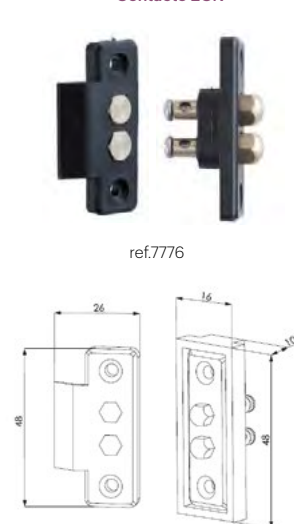
Contacto 2CN
