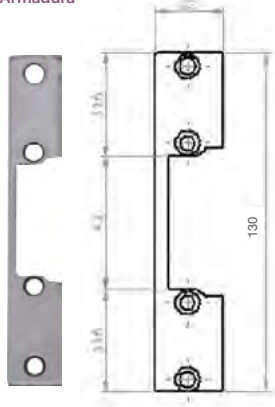
Armadura
